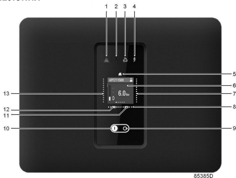
Панель управления
