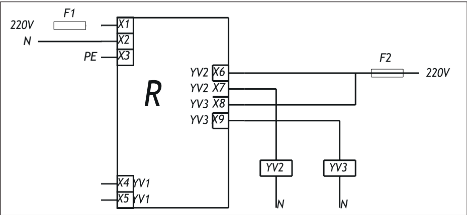
Abb.3.6.1. Elektroschaltplan
