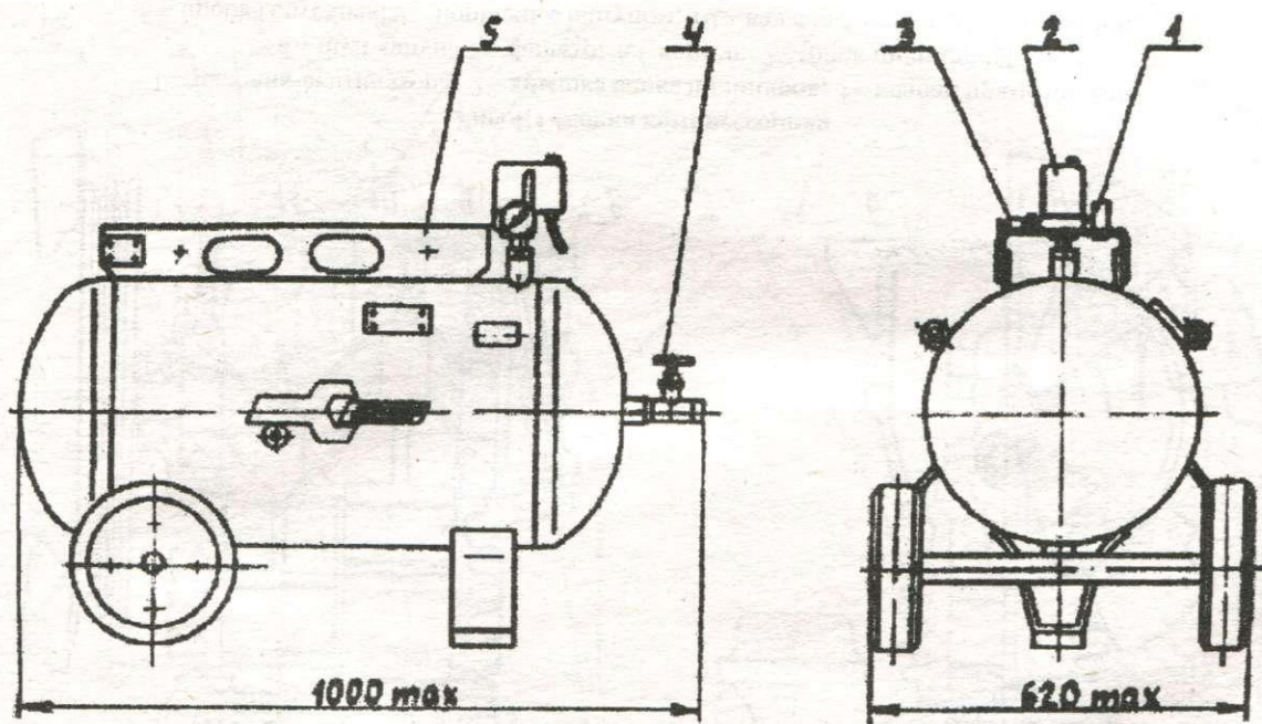
Рис. 5. Ресивер установки компрессорной, модель К-1, К-11, К-12, К-23 1 — манометр контроля воздуха; 2 — реле давления; 3 — клапан предохранительный; 4 — вентиль раздаточный; 5 — плита
