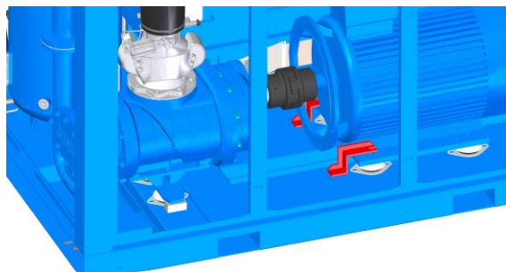
Рис. 25: Транспортный фиксатор
