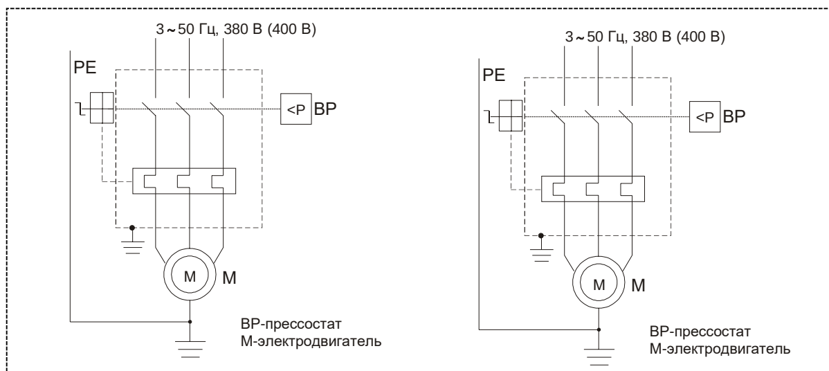
Рисунок А.2 – Схема электрическая принципиальная компрессора CB4/Ф-500.AB678TB
