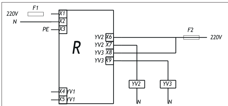
Abb.3.6.1. Elektroschaltplan
