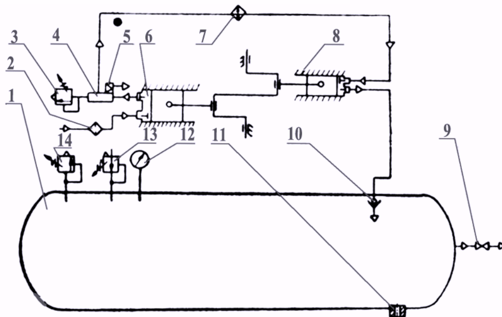
Рис. 30. Схема пневматическая принципиальная установки компрессорной, модель К-5
