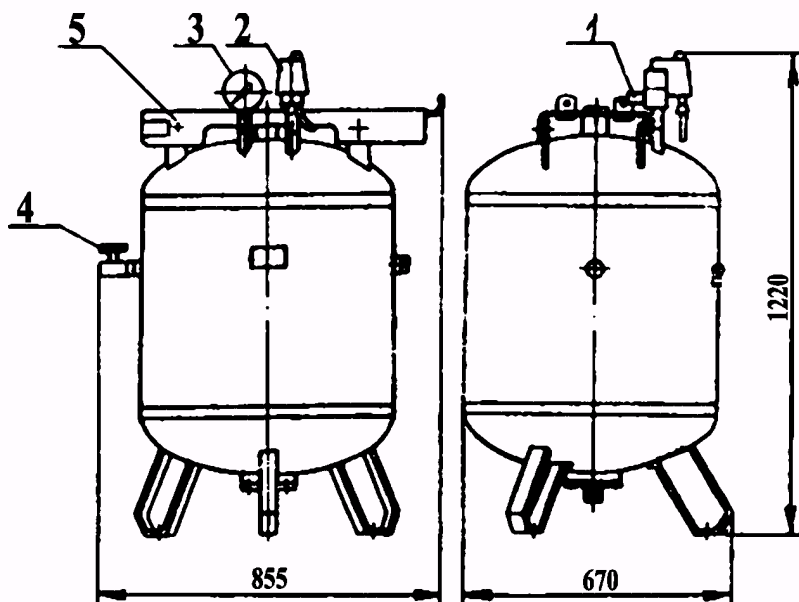
Рис. 21. Ресивер установки компрессорной, модель KB-15
